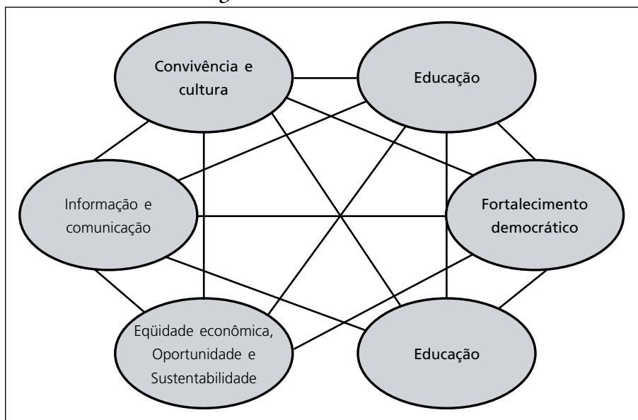
Figura 1. Valores Nucleares.
